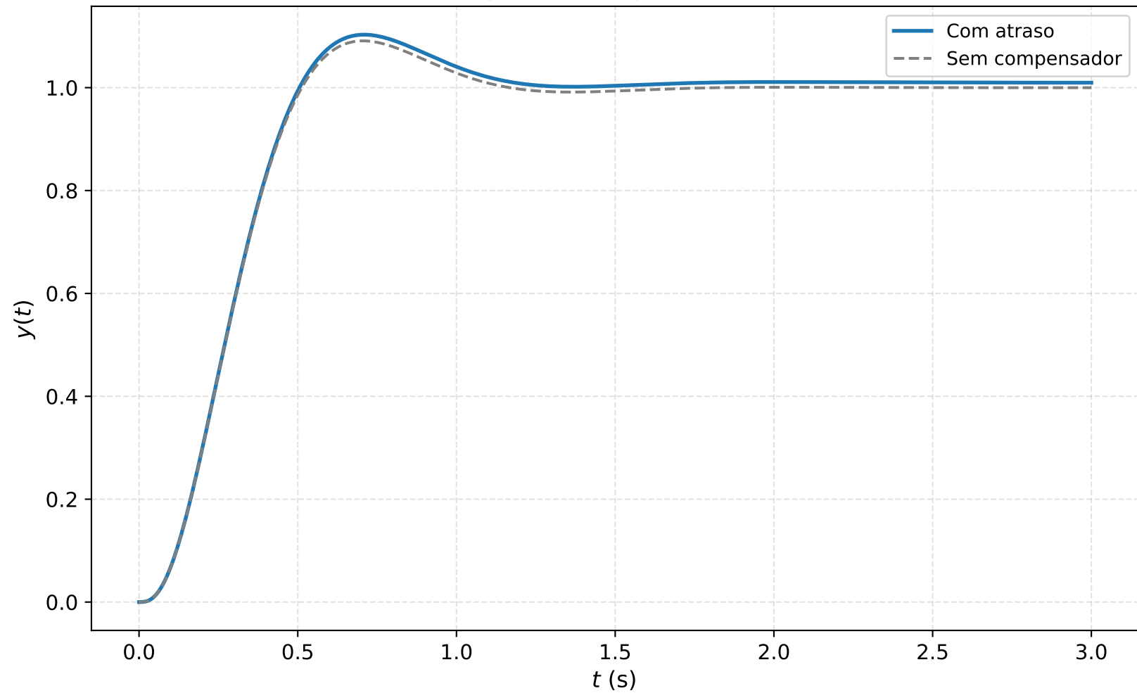
Resposta ao degrau unitário
